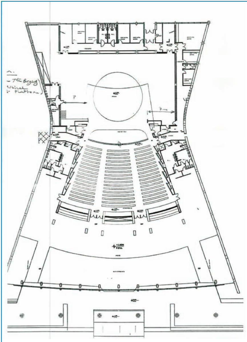
Echelle 1/300
